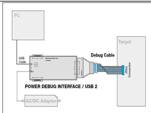
图 2.21 trace32 连接 PC 进行调试
