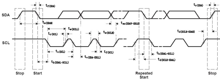
图 2.11 I2C 发送时序
