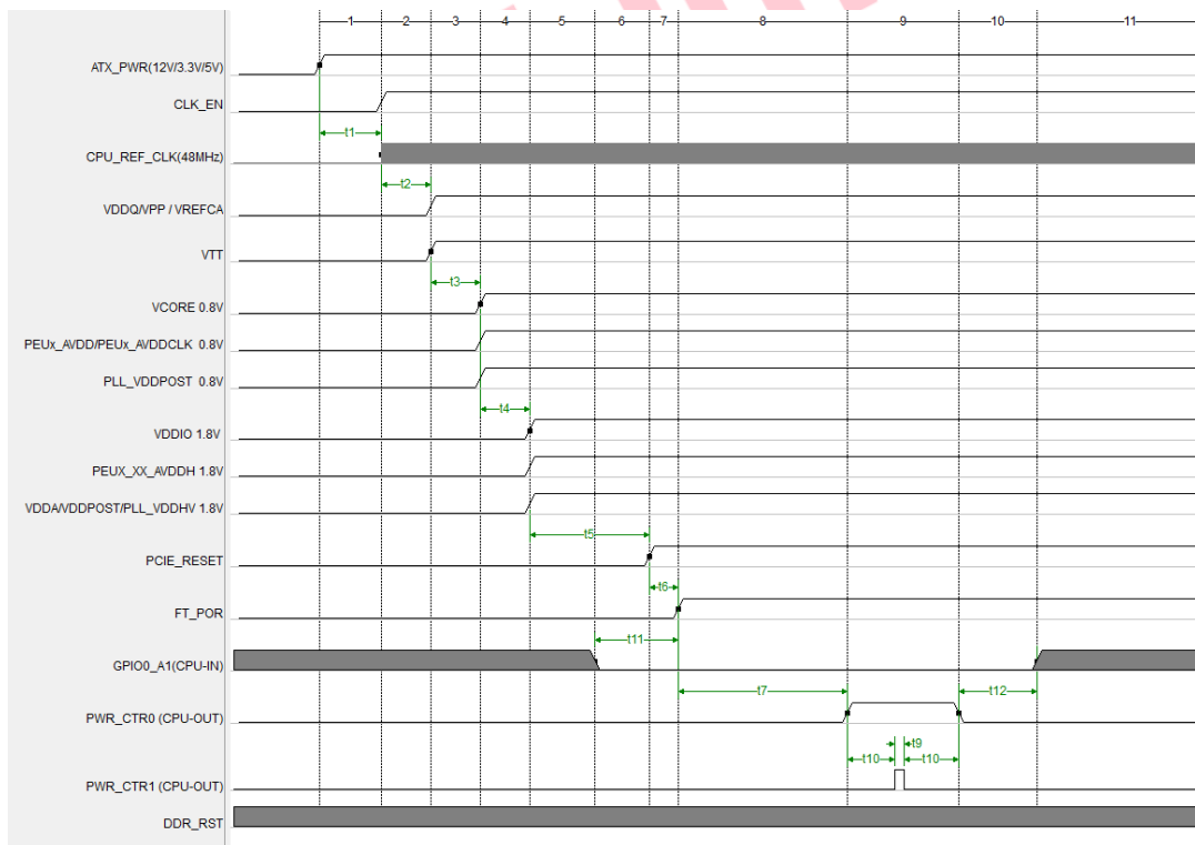
图 5.1 S4/S5→S0 开机时序图
