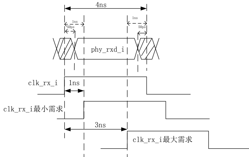
图 2.9 RX 数据端口采样时序图
