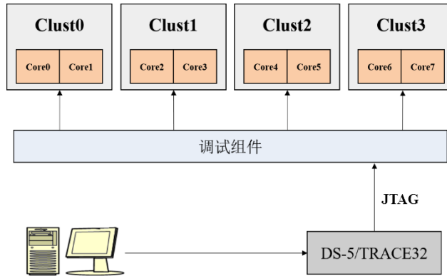
图 2.20 D2000 软件调试结构
