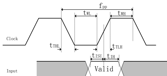
图 2.19 SD 卡时钟数据输入输出时序图（高速模式）
