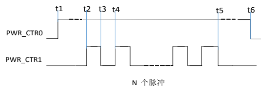
图 5.6 时序图
