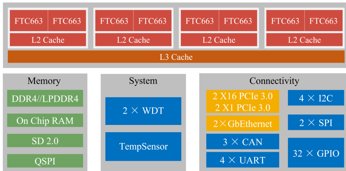
图 1.1 D2000 功能框图
