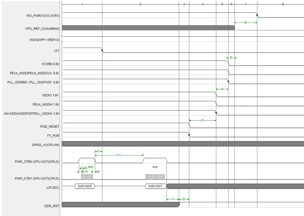
图 5.3 S0→S3 休眠时序图
