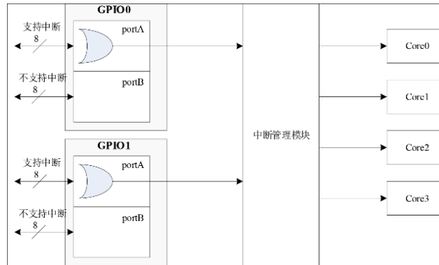
图 2.16 GPIO 中断结构图
