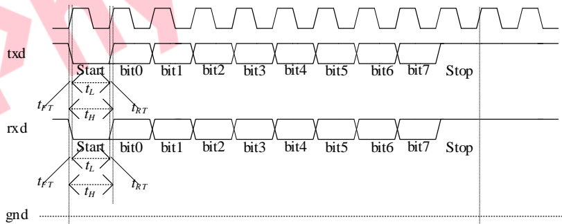
图 2.15 UART 时序图
