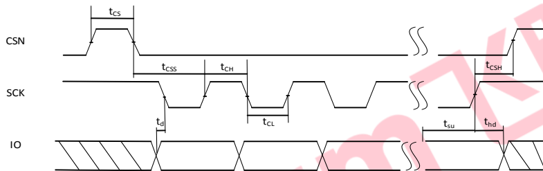
图 2.13 QSPI 总线时序
