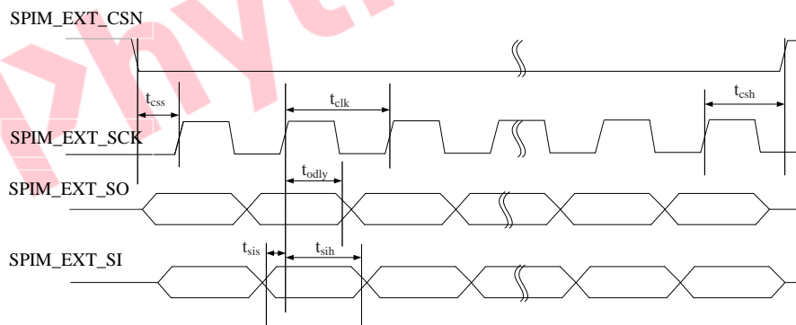
图 2.14 SPI 时序图
