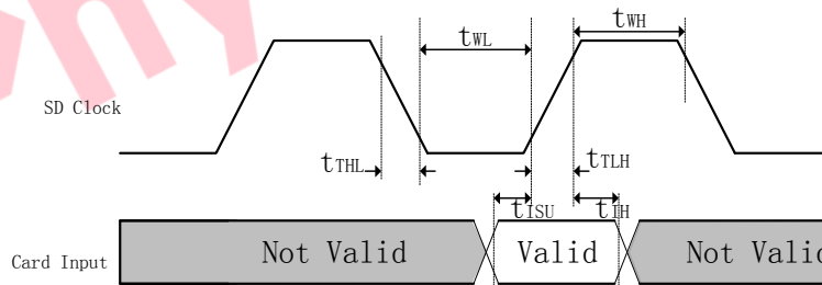
图 2.18 SD 卡时钟数据输入输出时序图 (标准模式)
