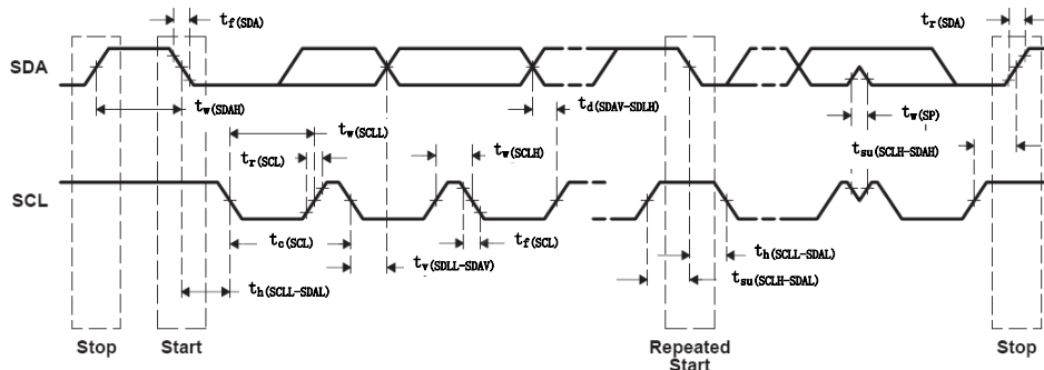
图 2.10 I2C 接收时序
