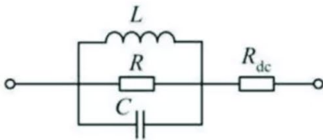
(c) 等效电路
