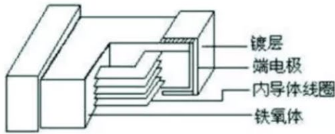
(b) 片式铁氧体磁珠的结构
